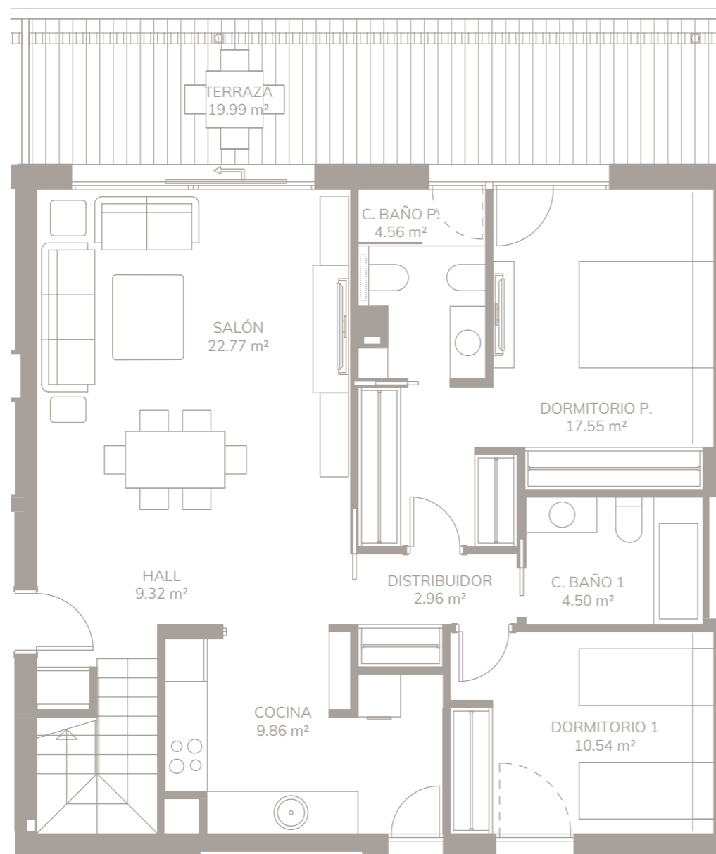
PLANTA ÁTICO
